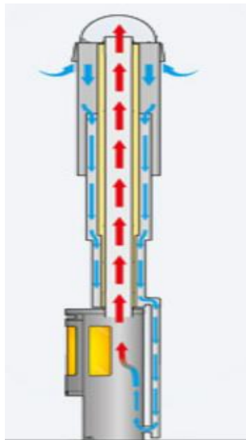
Figur 1 Illustrasjon av hvordan tilluftsrør fungerer
